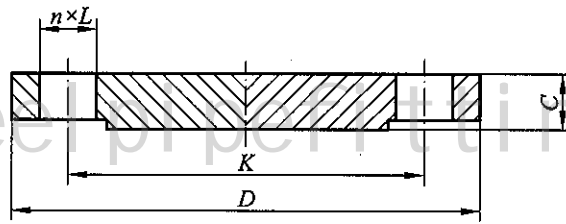
图 8.2.9 钢制管法兰盖 表 8.2.9-1 PN2.5 钢制管法兰盖
