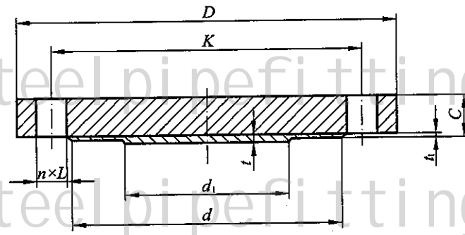
突面 (RF)
