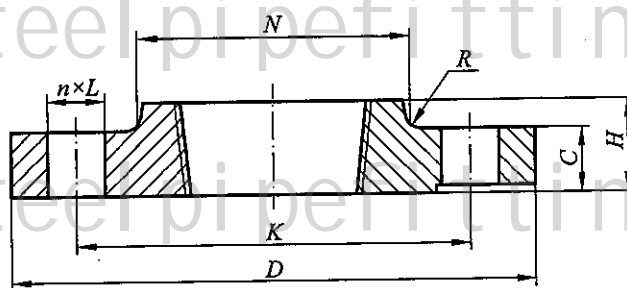
图 8.2.6 螺纹钢制管法兰
