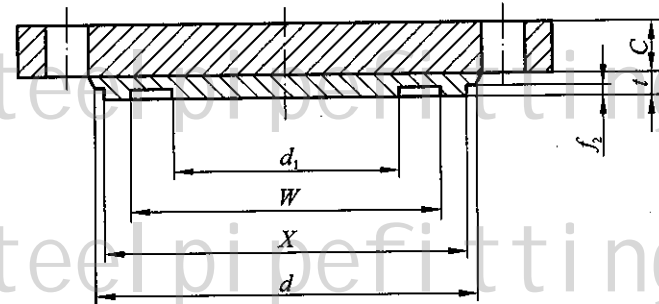
榫面 (T)
