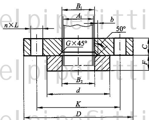
图 8.2.8 平焊环松套钢制管法兰
