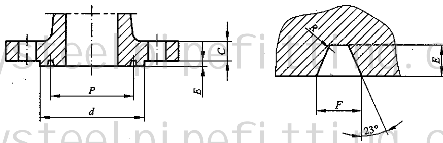
图 3.2.5-2 环连接面的密封面尺寸
